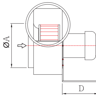
TYPE-FSM 尺寸表
