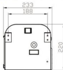
尺寸圖：單位mm
